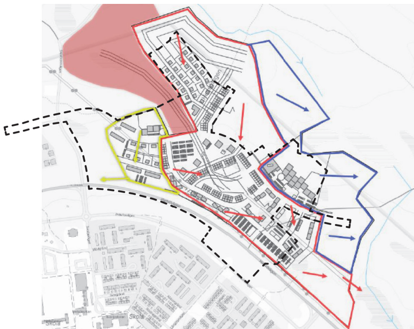
Figur 10. Områdesindelning för översiktlig princip för dagvattenhanteringen. Gult område leds västerut, rött område leds till tvåstegsdike och blått område leds till naturmark. Svart streckad linje visar ungefärlig avgränsning för planområdet.
